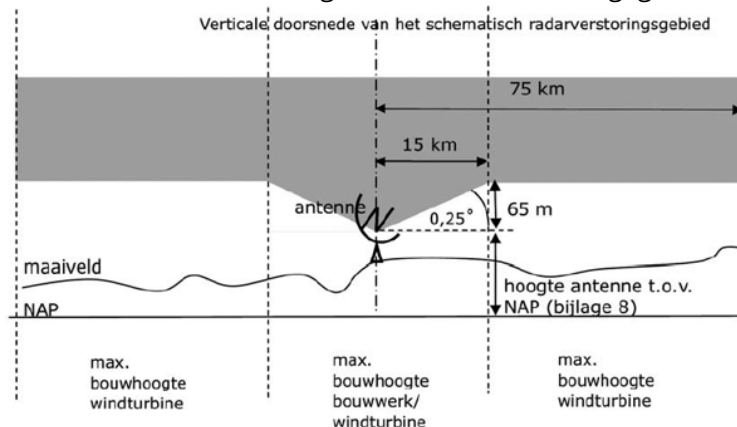
Schematische weergave bouwhoogte i.r.t. radarverstoring
