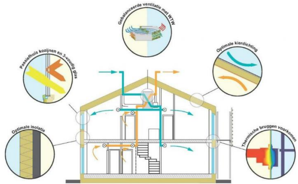
Bouwkundige kenmerken van de passieve bouwwijze Toegepast op een compact ontwerp met de juiste oriëntatie
